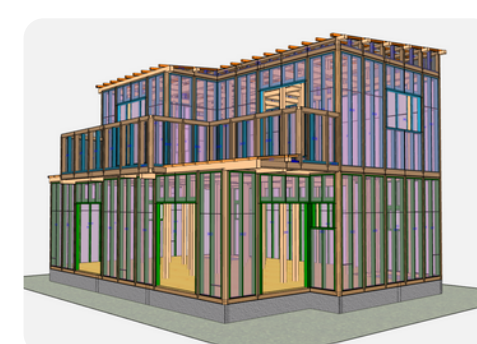
軸組パネルデータ作成
